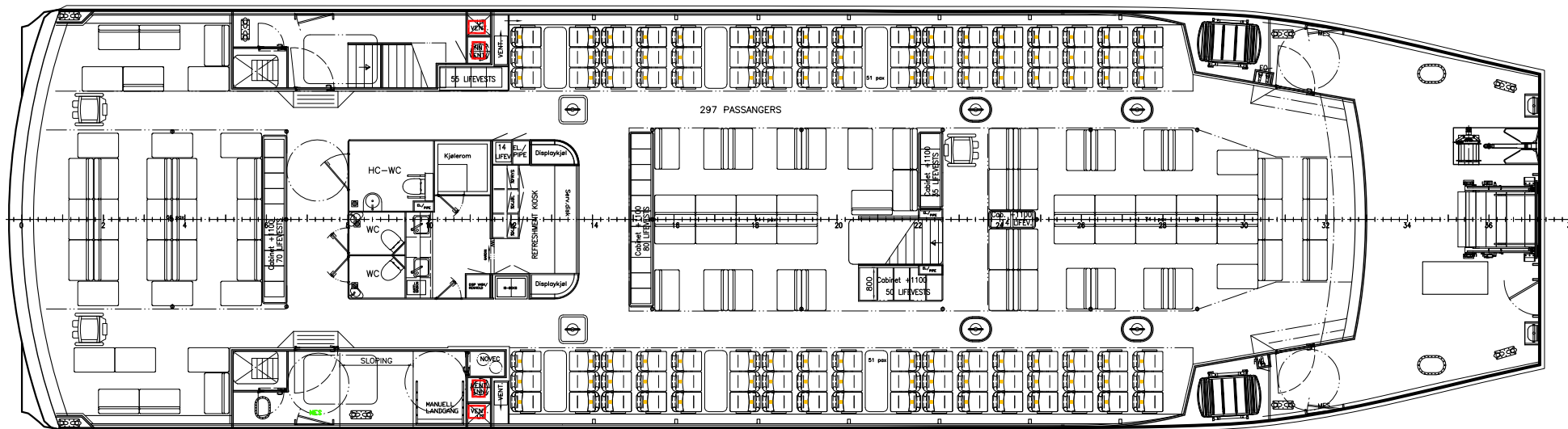
PLAN MAIN DECK (SOMMER SIGHTSEEING PRODUKSJON)
