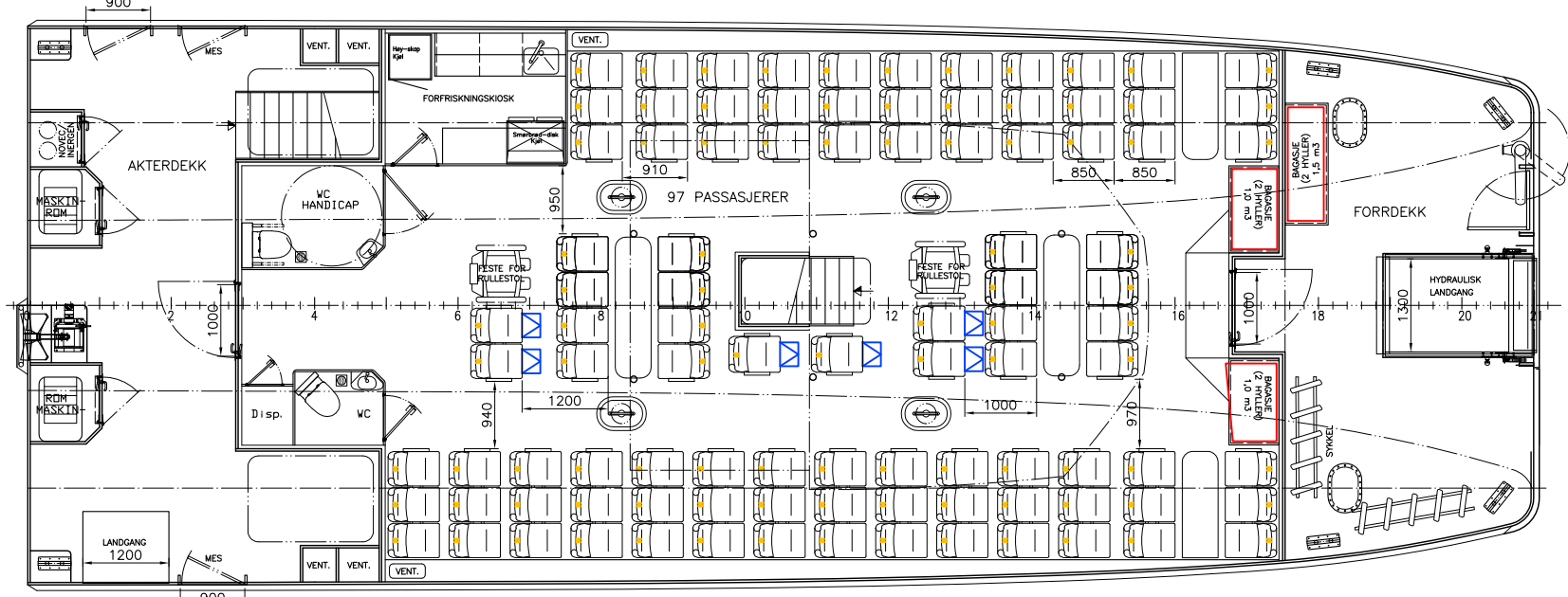
HOVEDDEKK OG BRO
