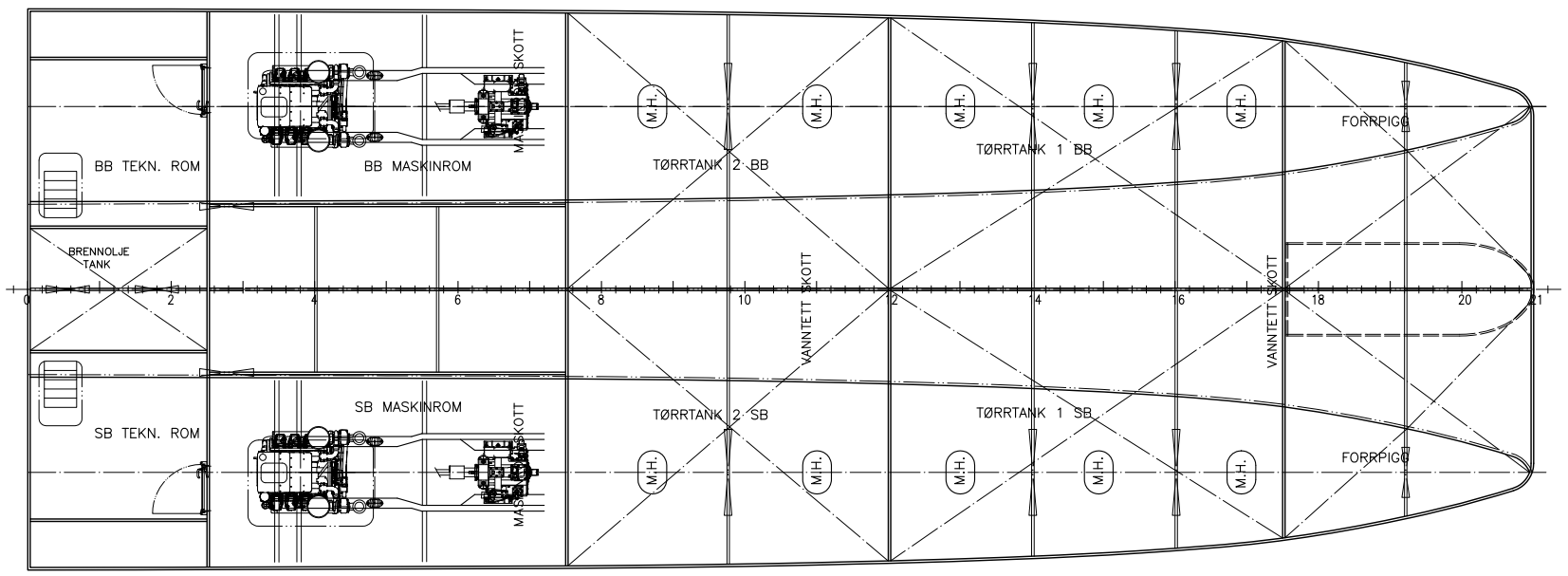
PLAN UNDER HOVEDDEKK
