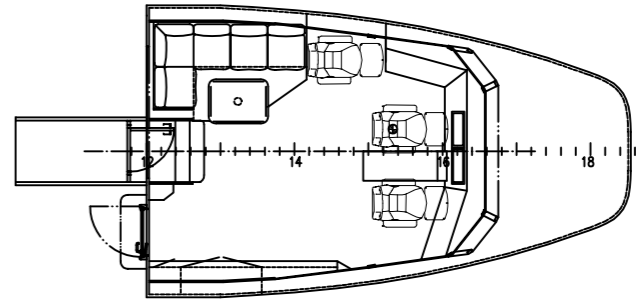
PLAN STYREHUS
