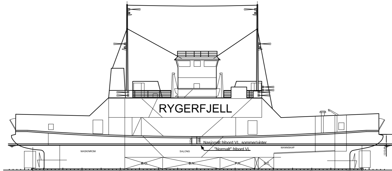
PROFIL
