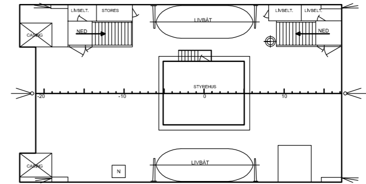
REPOSDEKK
