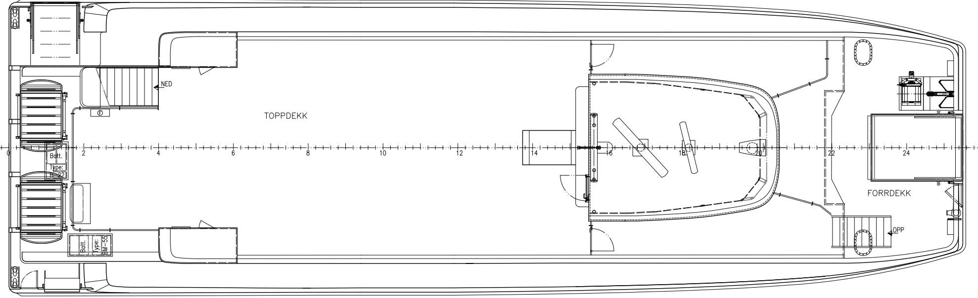
UTVENDIGE DEKK
