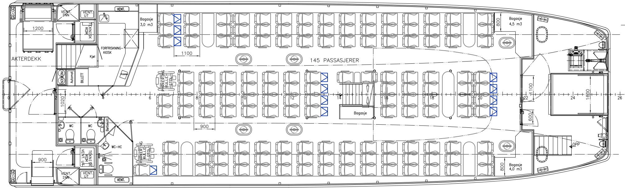
PLAN HOVEDDEKK
